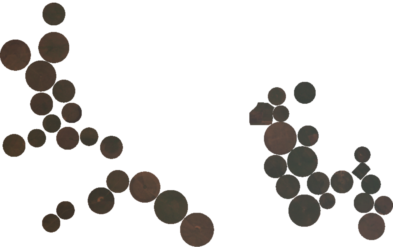
RGB map 40
