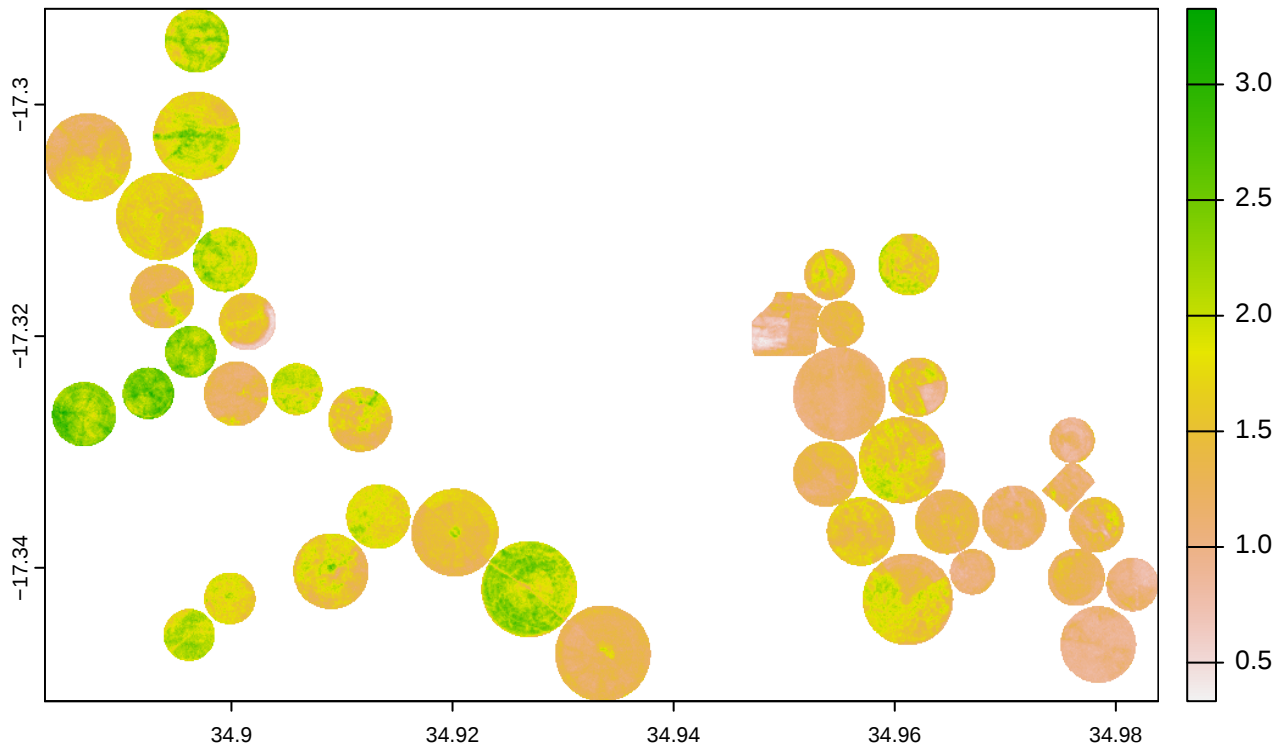
CI map 40
